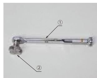
① トルクレンチ (N900QLK) FAS-001-0171 ② ヘッド治具 (SUS) JP-20168
